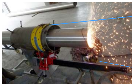
爪钉式套管工装
